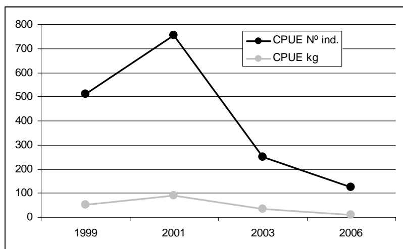
Figura I.4.: Captura por unidad de esfuerzo en número (CPUE n° ) y captura por unidad de esfuerzo en kg. (CPUE Kg) para los años 1999, 2001, 2003 y 2006 en la laguna El Cuerú.
