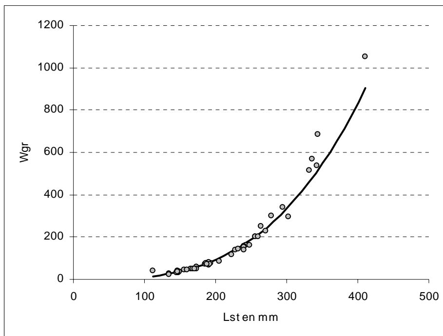
Figura I.6.: Relación entre la longitud y el peso de los pejerreyes capturados en la laguna El Cuerú, en círculos valores observados, en línea modelo ajustado.
