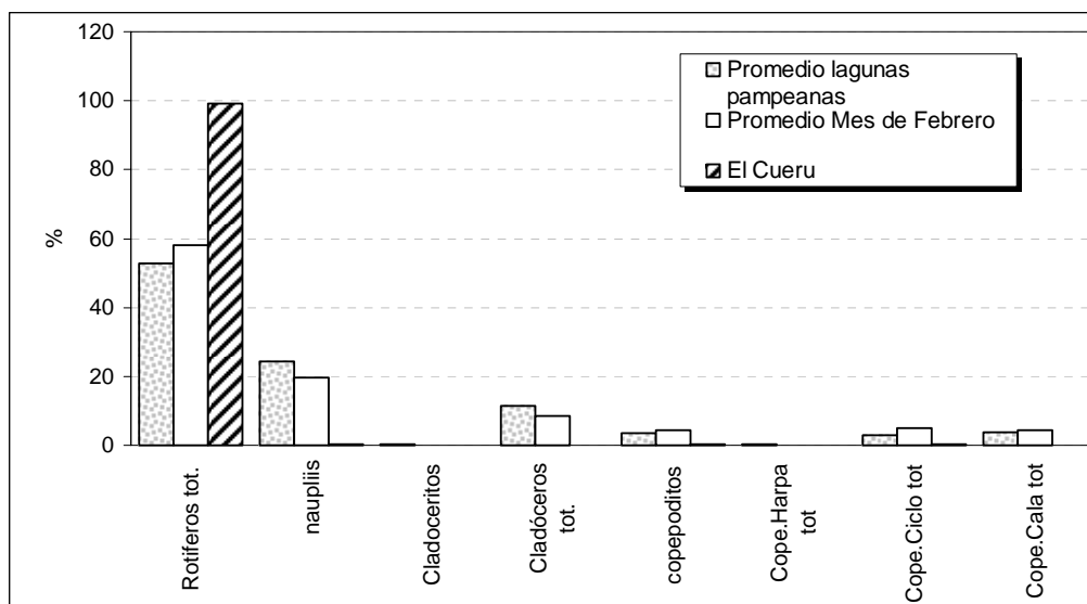
Figura Z.1: Abundancia relativa de los principales grupos zooplanctónicos en la laguna El Cuerú.
