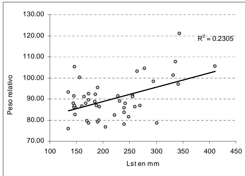
Figura I.5.: Peso relativo promedio (Wr.) obtenido en función de la longitud estándar (Lst.) de los pejerreyes capturados en la laguna El Cuerú.
