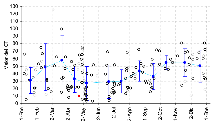
Figura 2P: Valores correspondientes al ICT obtenido para diferentes fechas en los ambientes estudiados dentro de la provincia de Buenos Aires. Los puntos azules representan los valores promedio para cada mes y el punto rojo corresponde al cuerpo de agua en cuestión.
