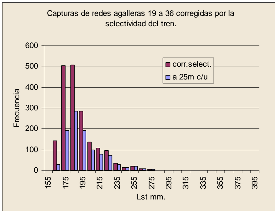
Figura 2I distribución de tallas estimada para una longitud de 25 m para los paños 19 a 36 (azul) corrección de la distribución por la selectividad de las respectivas redes (marron).
