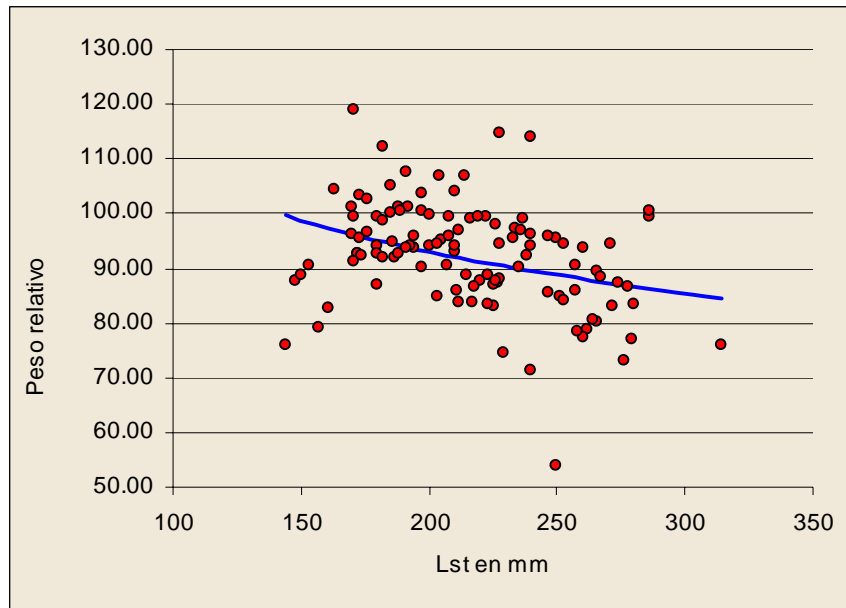
Figura 4I: Peso relativo promedio (Wr.) obtenido en función de la longitud estándar (Lst.) de los pejerreyes capturados en la laguna La tigua.
