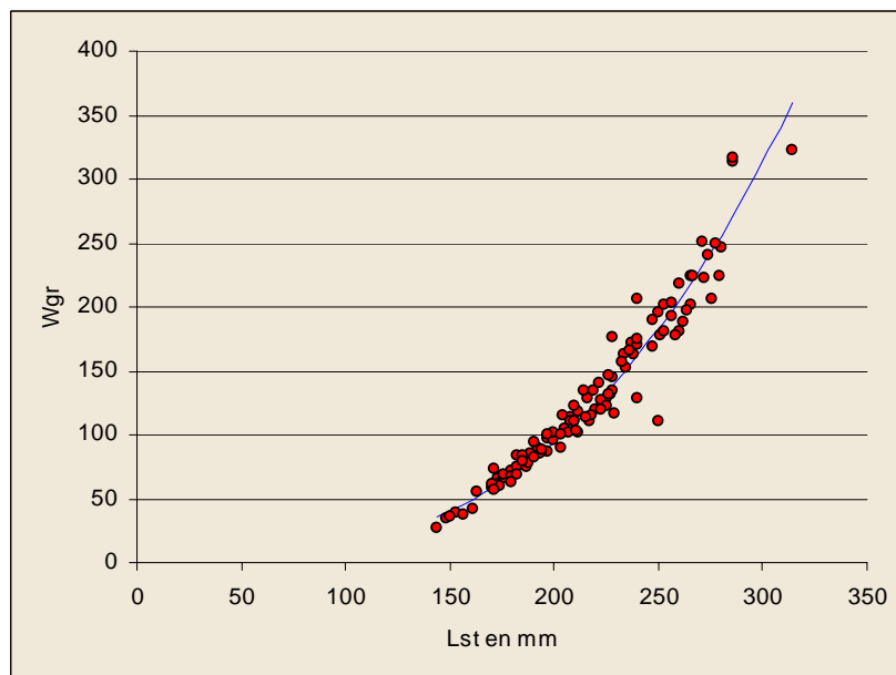
Figura 5I: Relación entre la longitud y el peso de los pejerreyes capturados en la laguna La tigua, en puntos rojos valores observados, en línea azul modelo ajustado.
