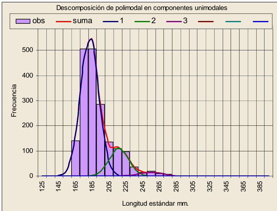
Figura 3I Descomposición de la distribución multimodal de tallas corregida por la selectividad de las redes agalleras en sus componentes unimodales
