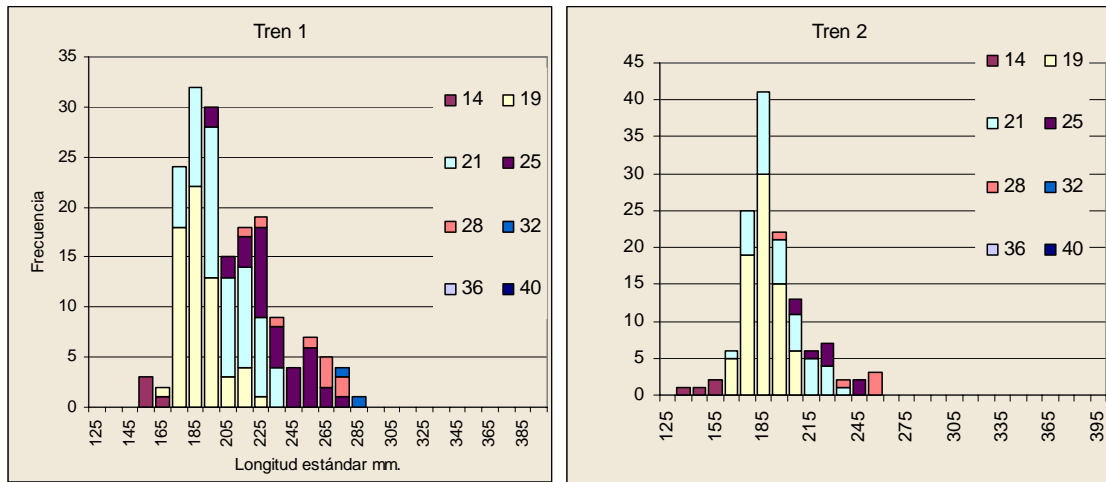
Figura 1I: Distribución de las capturas totales ordenadas cada intervalos de 10mm de longitud estándar (Lst.).
