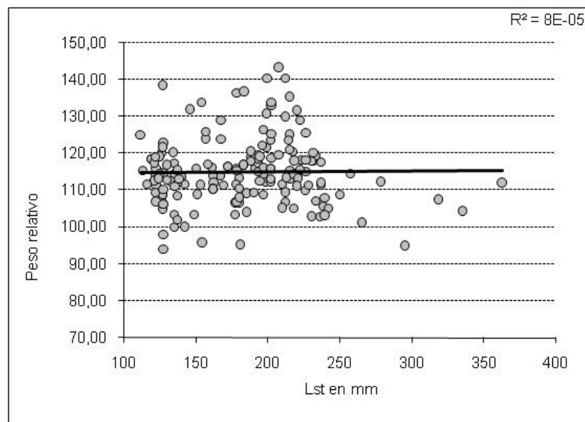
Figura 12: Peso relativo promedio ( W_r ) obtenido en función de la longitud estándar (Lst.) de los pejerreyes capturados en la laguna Gómez.
