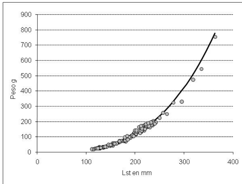
Figura 13: Relación entre la longitud y el peso de los pejerreyes capturados en la laguna Gómez, en círculos valores observados, en línea modelo ajustado.
