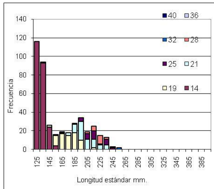
Figura 7: Distribución de las capturas totales ordenadas cada intervalos de 10mm de longitud estándar (Lst.) para cada uno de los trenes.
