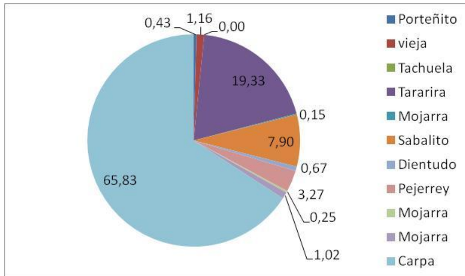
Figura 4: Abundancia relativa promedio de la biomasa de las especies capturas en la laguna Gómez con trampas.
