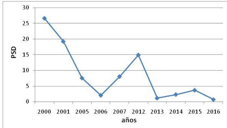
Figura 10. PSD para la población de pejerrey de la laguna Gómez.
