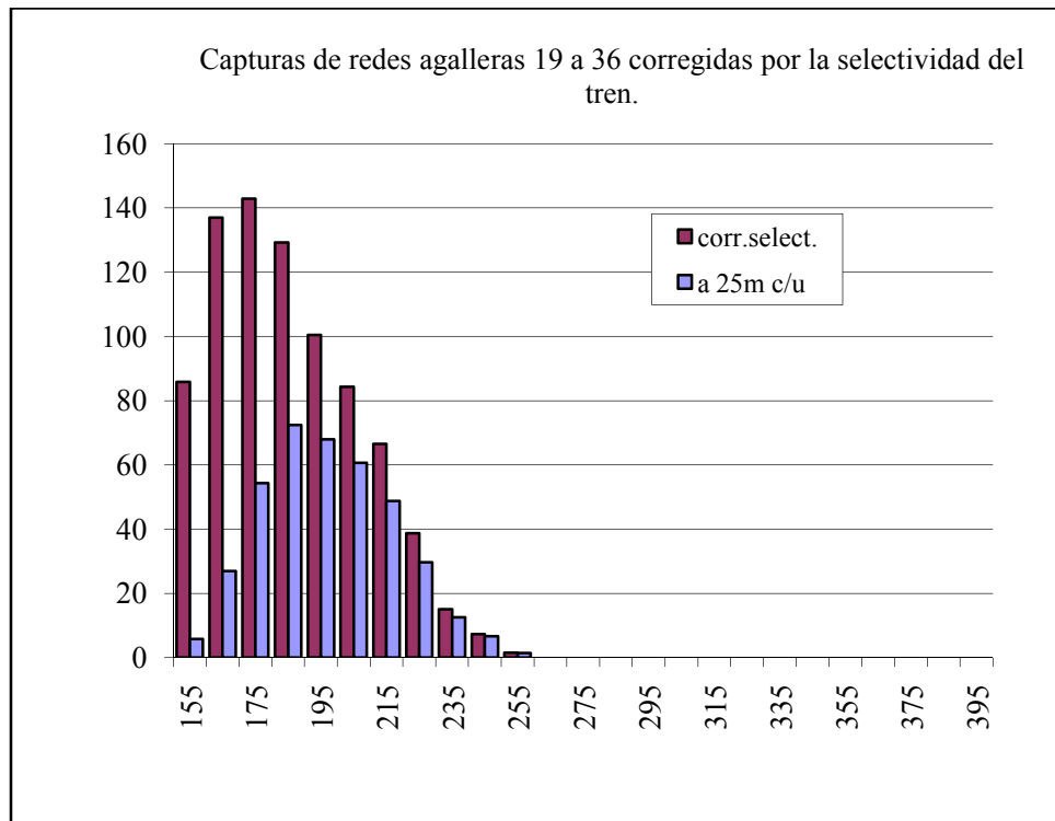
Figura 7: Distribución de tallas estimada para una longitud de 25 m para los paños 19 a 36 y corrección de la distribución por la selectividad de las respectivas redes.
