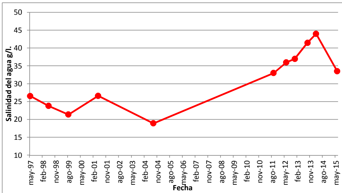
Figura 8: Salinidad del agua de la laguna Chasicó durante 1997, 1998, 1999, 2001, 2004, 2011, 2012, 2013, 2014 y 2015.
