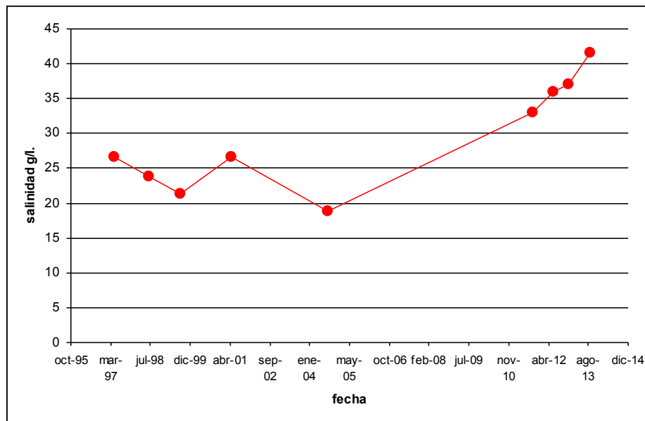
Figura 8.: Salinidad del agua de la laguna Chasicó durante 1997, 1998, 1999, 2001, 2004, 2011 y 2012.
