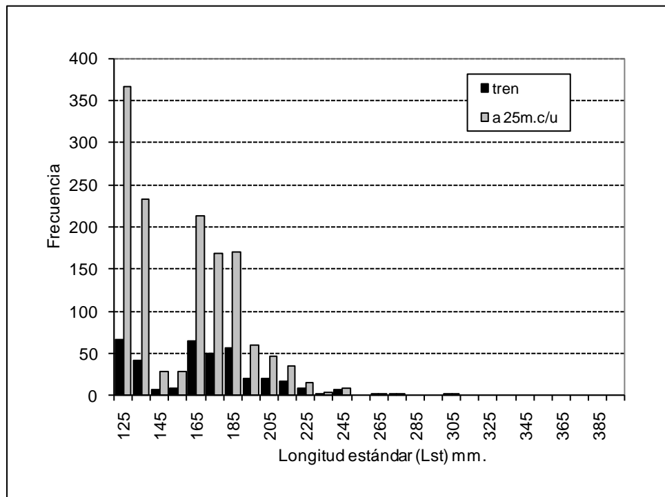
Figura I. 2.: Distribución de tallas de capturas totales de los dos trenes y transformada a una longitud de 25 m para todos los paños para la laguna de Saavedra.
