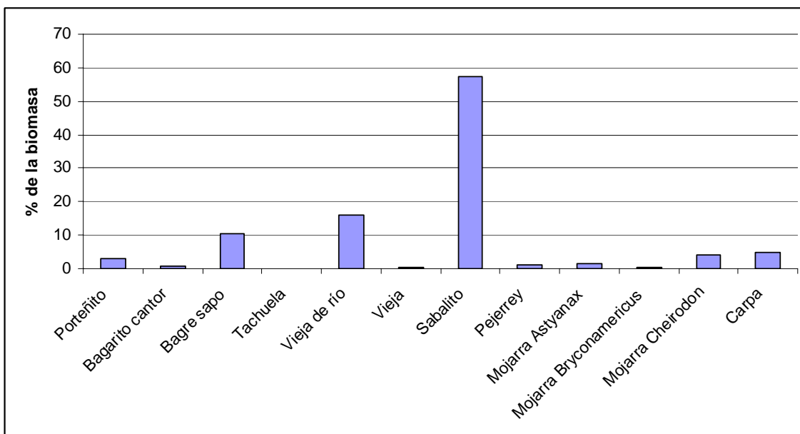
Figura I.3: Abundancia relativa promedio de la biomasa de las especies capturas en la laguna Lobos.
