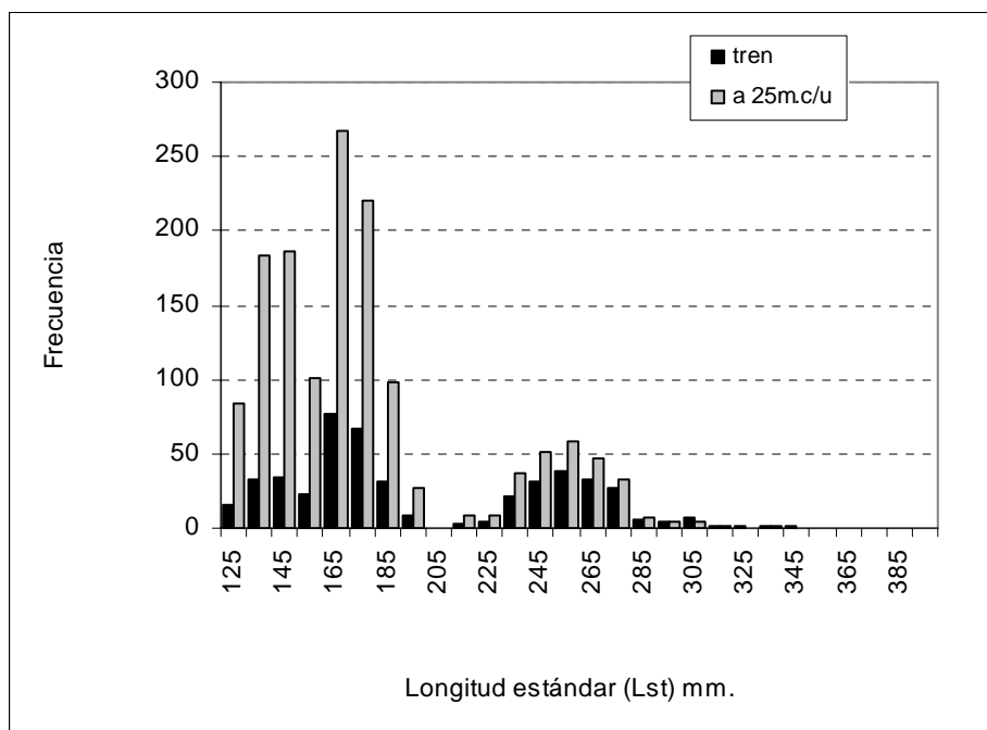
Figura I. 5.: Distribución de tallas de capturas totales de los dos trenes y transformada a una longitud de 25 m para todos los paños para la laguna Lobos.
