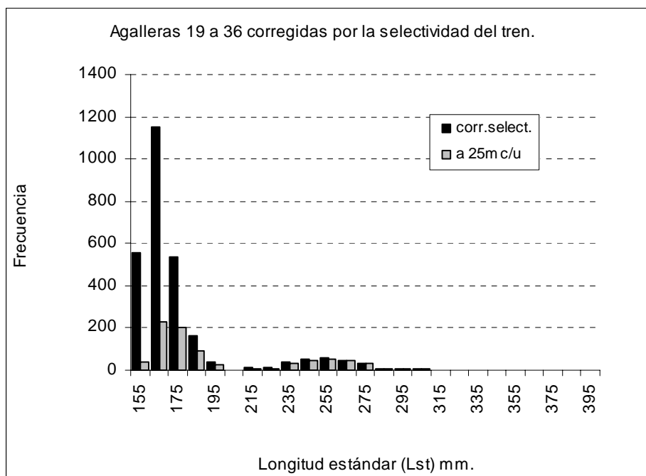
Figura I.6. Distribución de tallas estimada para una longitud de 25 m para los paños 19 a 36 y corrección de la distribución por la selectividad de las respectivas redes para la laguna Lobos.
