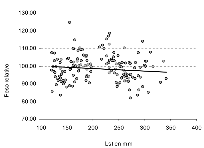
Figura I.10.: Peso relativo promedio (Wr.) obtenido en función de la longitud estándar (Lst.) de los pejerreyes capturados en la laguna Lobos.
