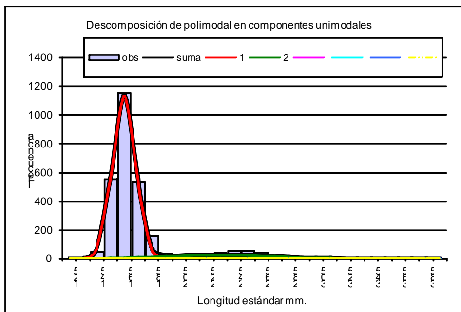
Figura I.7: Descomposición de la distribución polimodal de tallas corregida por la selectividad de las redes agalleras en sus componentes unimodales
