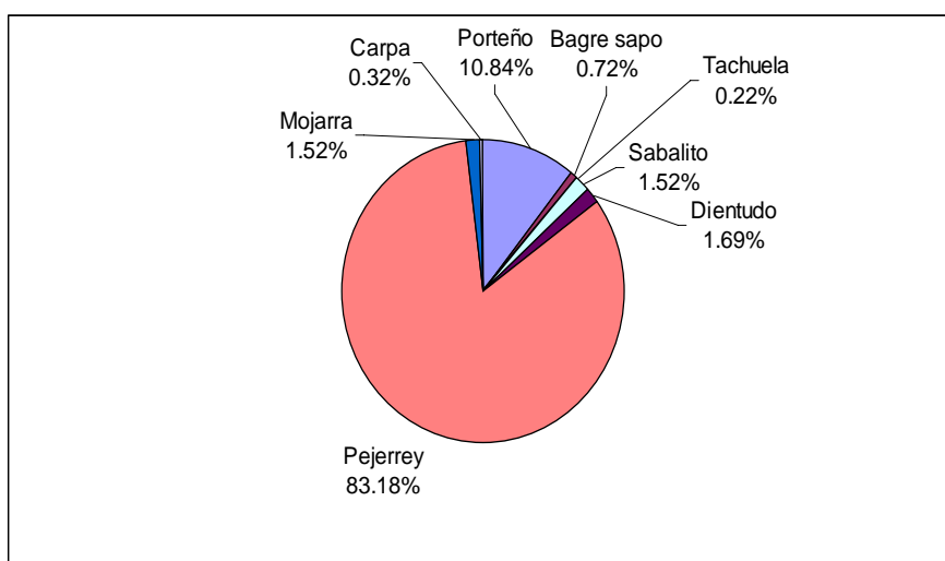
Figura I.1: Abundancia de las especies capturas con redes de enmalle en la laguna Lobos.
