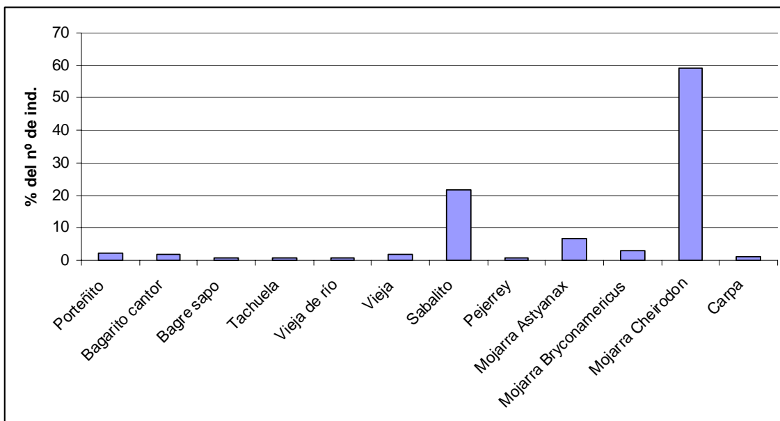
Figura I.2: Abundancia relativa promedio de las especies capturas en la laguna Lobos.
