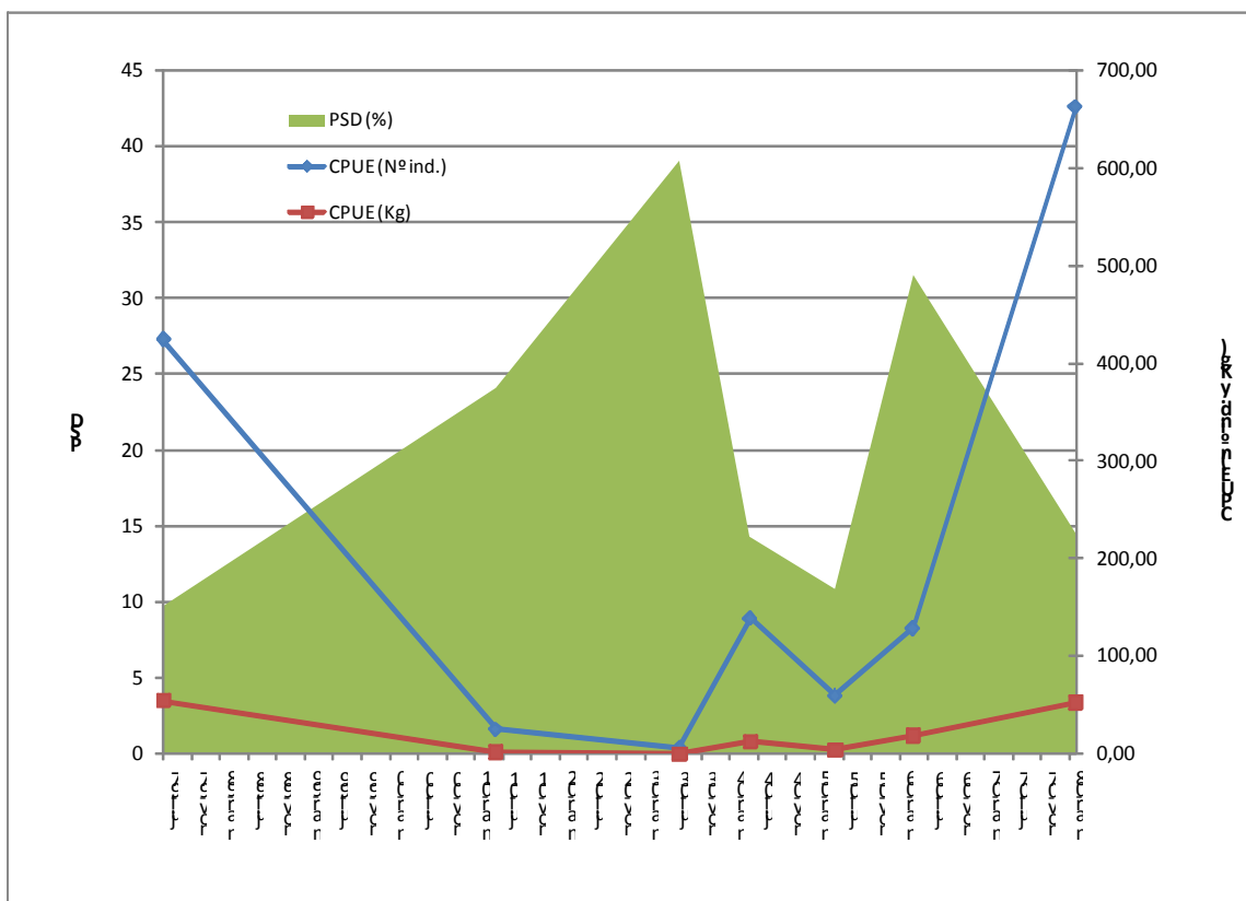
Figura I.9: Captura por unidad de esfuerzo en número (CPUE o ) y captura por unidad de esfuerzo en kg. (CPUE Kg) para los años 1997, 2001, 2003, 2004, 2005, 2006 y 2008 en la laguna Lobos.
