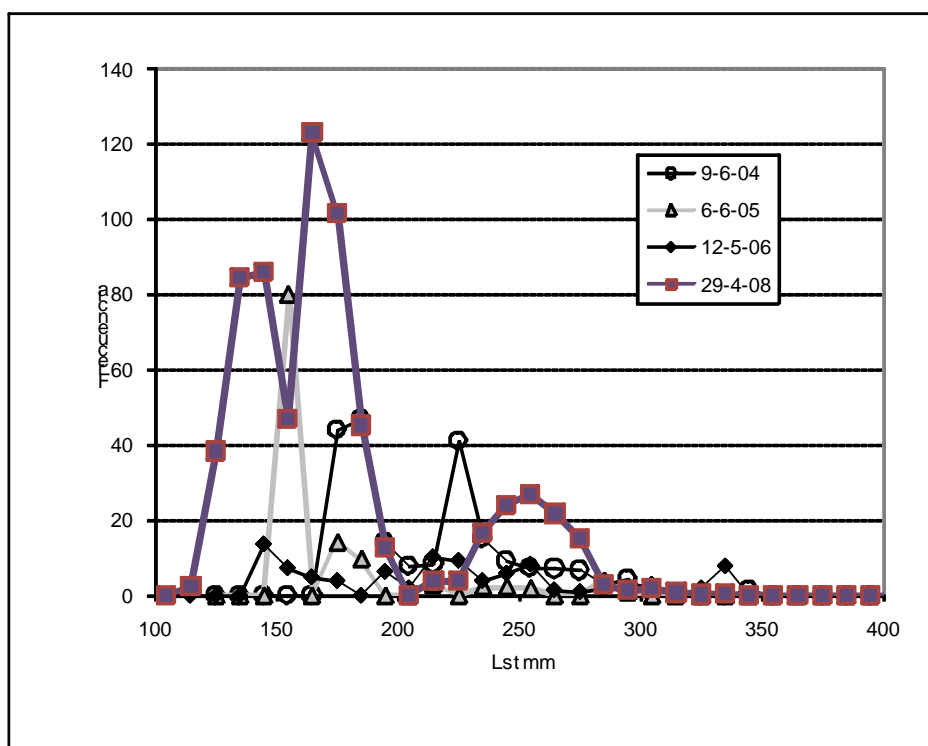
Figura I.8.: Distribución de tallas estimada corregida por la selectividad de las respectivas redes para los años 2004, 2005, 2006 y 2008 en la laguna Lobos.
